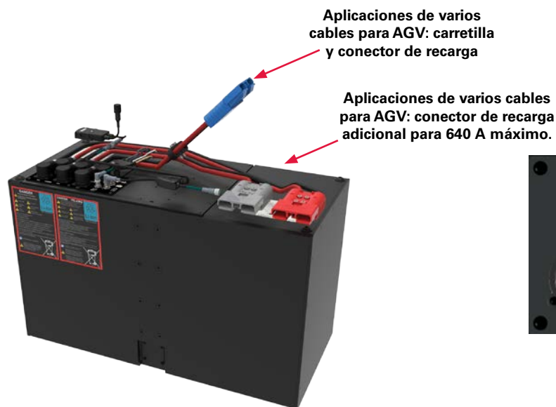
Figura 5: Aplicación de varios cables AGV
